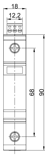
Габаритные размеры
